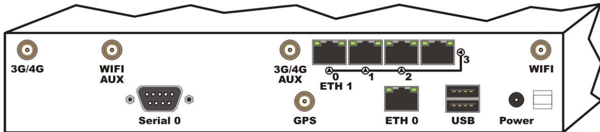
Abbildung 2: Rückseite ELW Router
